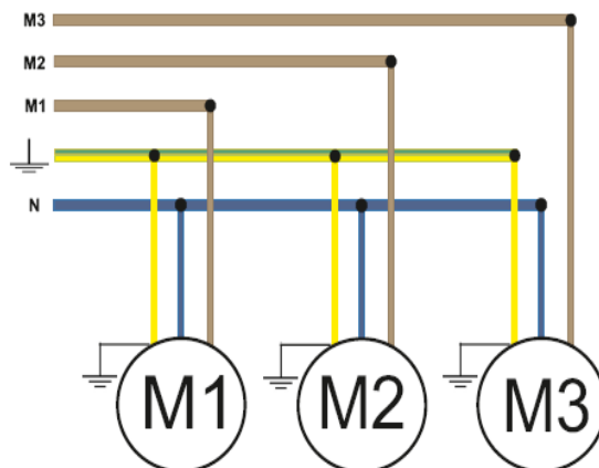
Figura 9: schema elettrico
