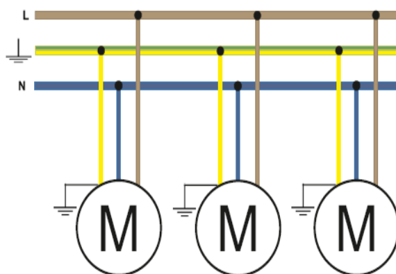
Figura 7: schema elettrico
