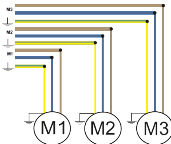
Figura 11: schema elettrico
